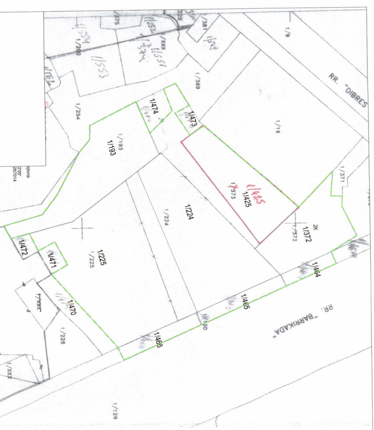
PLANI I VENDOSJES SË STRUKTURËS SHK. 1:200
