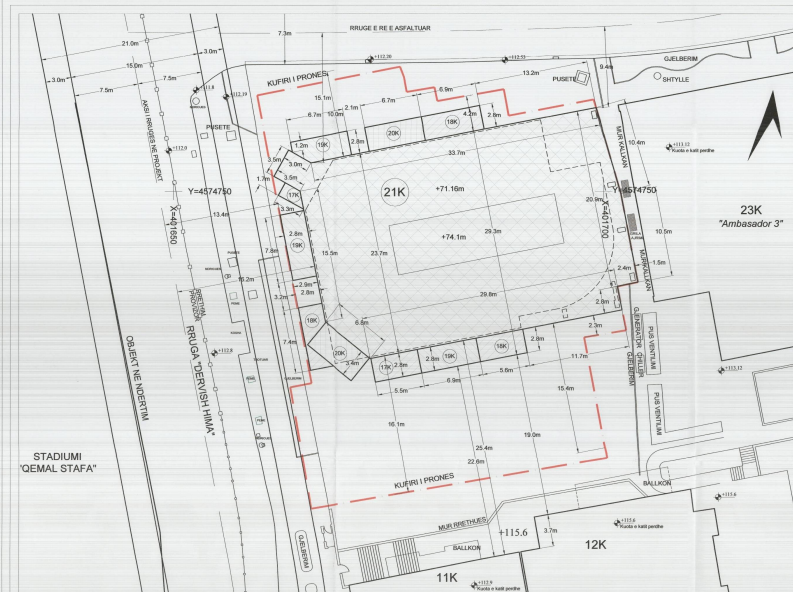
PLANI I VENDOSJES SË STRUKTURËS SHK. 1: 200
